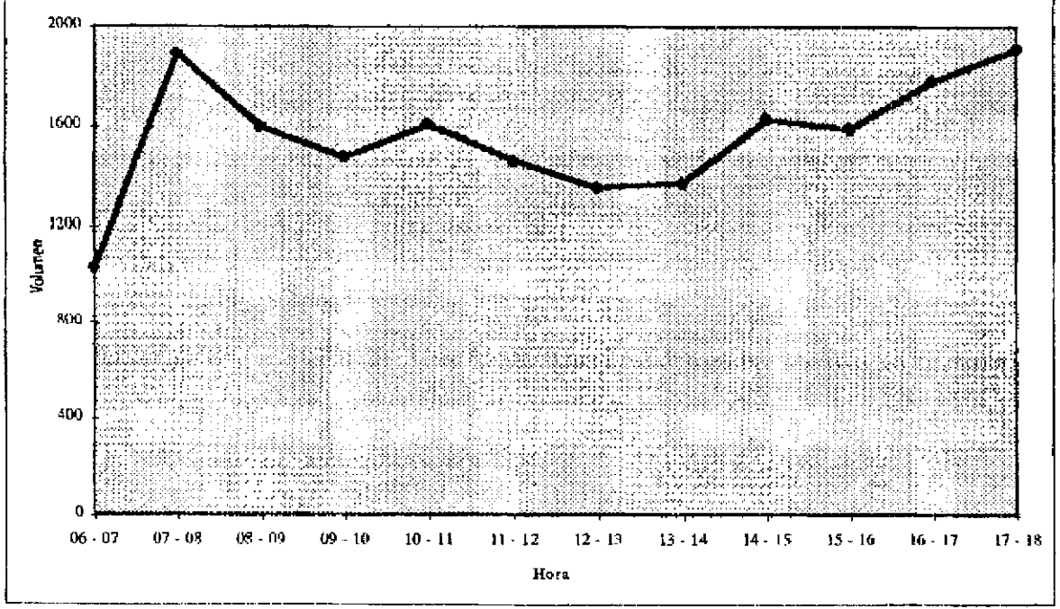
FIGURA 10 Perfil de Variación Horaria Ruta 3
