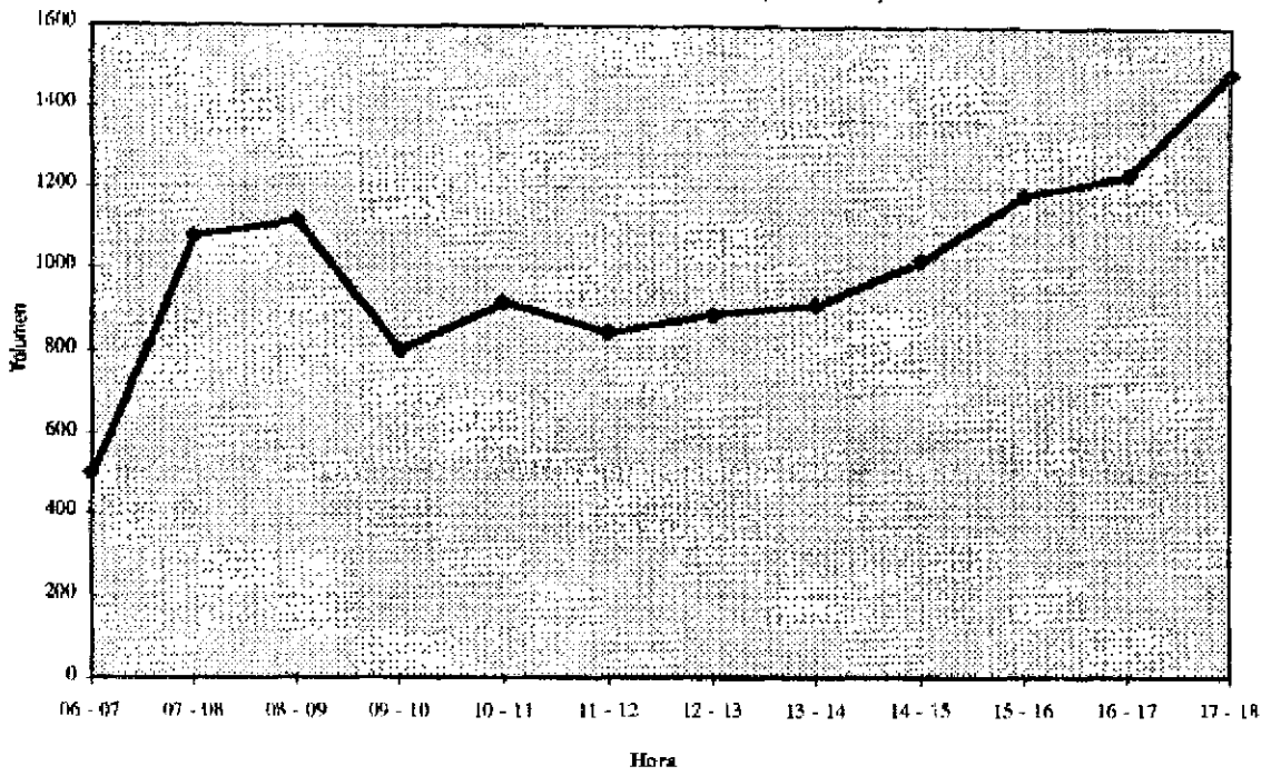
FIGURA 11 Perfil de Variación Horaria Ruta 27 (Santa Ana)
