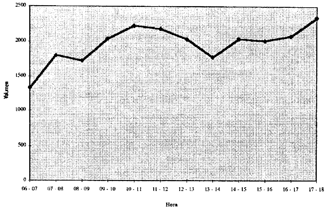
FIGURA 5 Perfil de Variación Horaria Ruta 2 (San Pedro)
