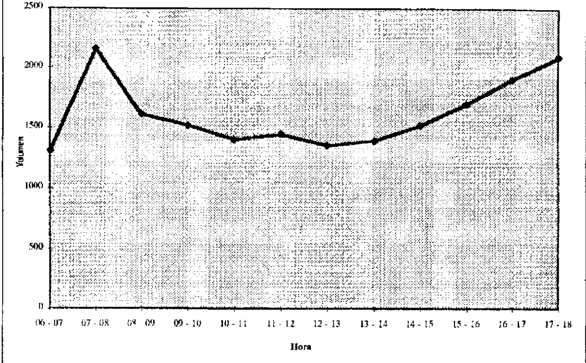
FIGURA 9 Perfil de Variación Horaria Ruta 2 (Antes Cartago)
