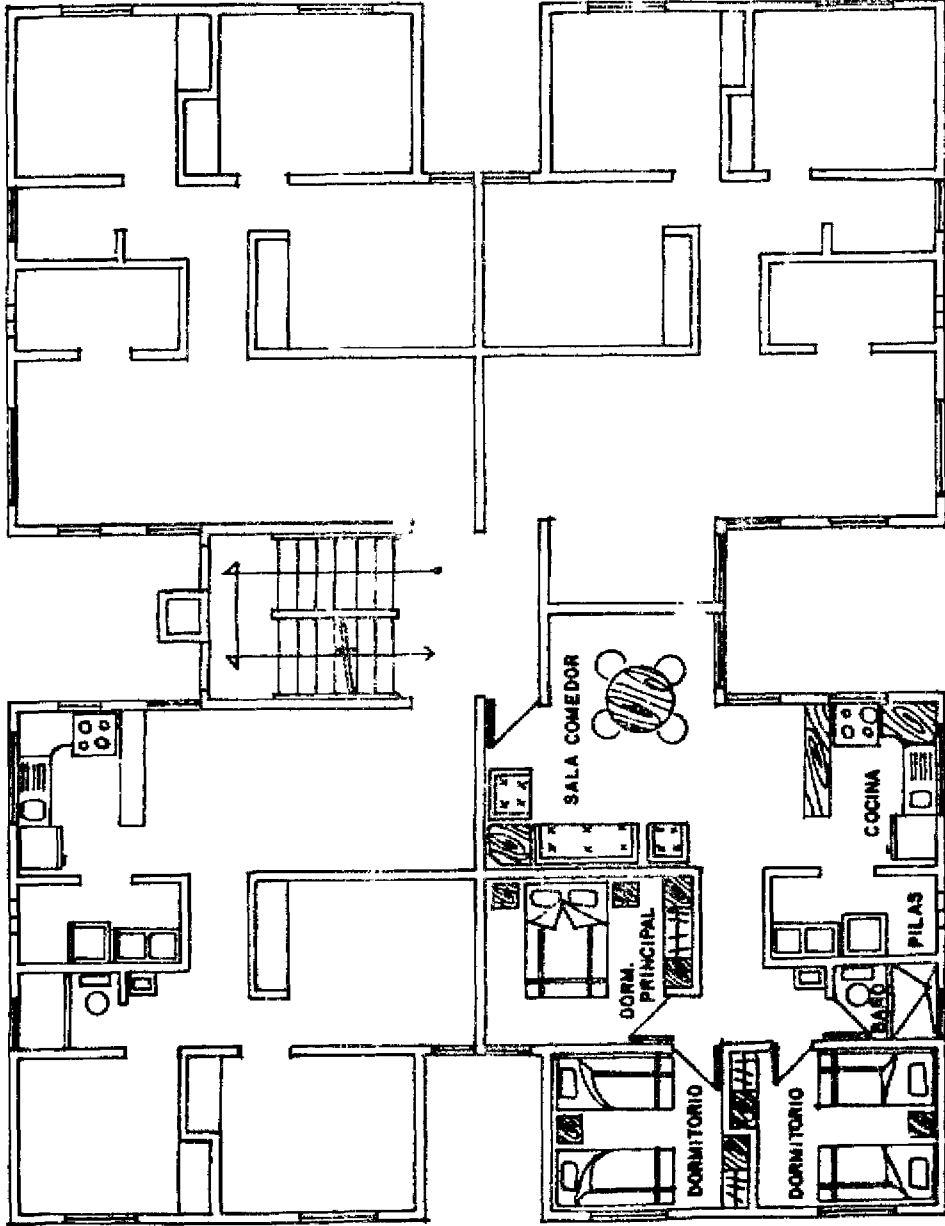
PLANTA GENERAL EDIFICIO TIPO R045 SOLUCION B45E.
