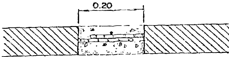
JUNTA HORIZONTAL ENTRE LOSAS DE ENTREPISO
