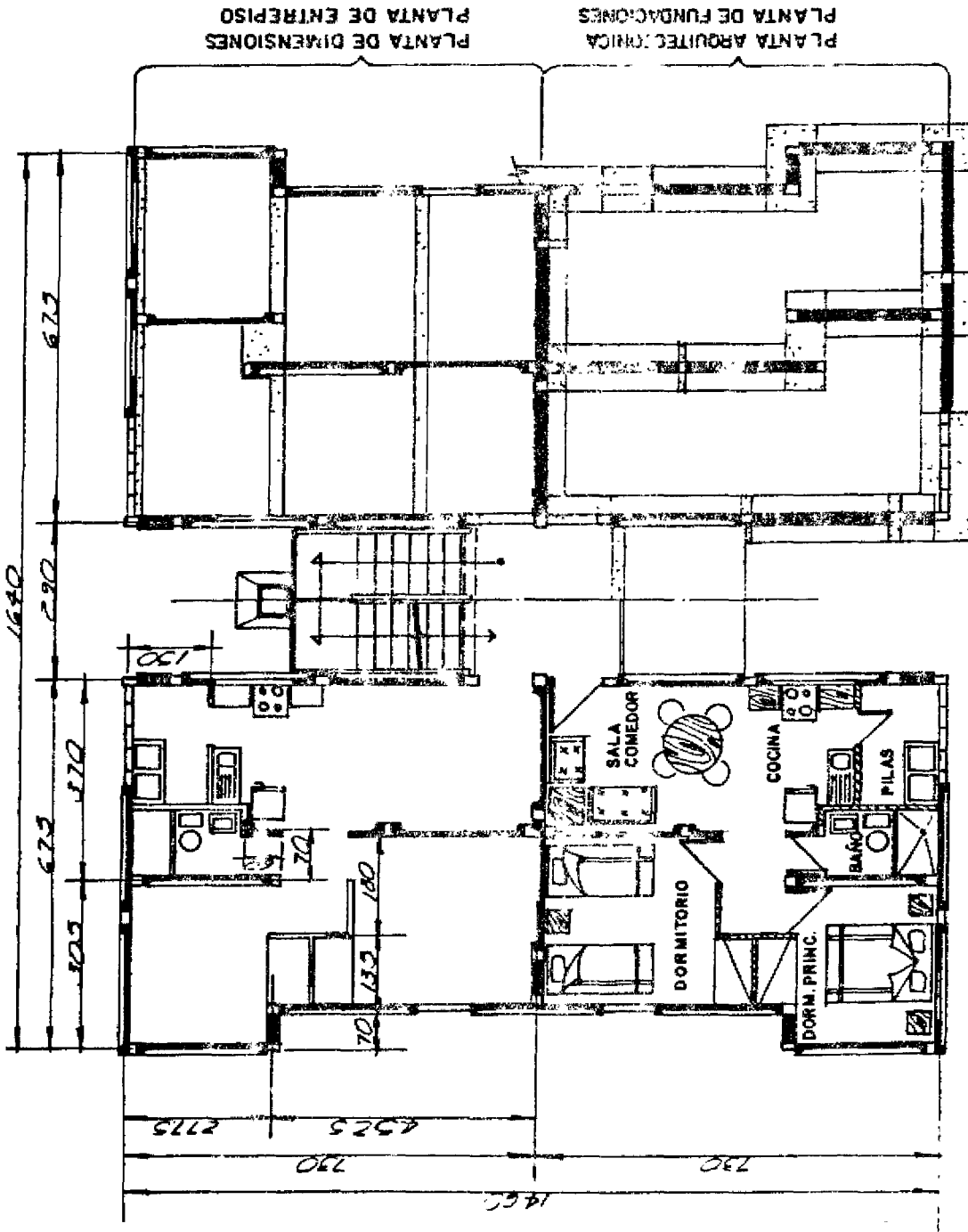
PLANTA GENERAL EDIFICIO TIPO IRAZU SOLUCION PREFABRICADA
