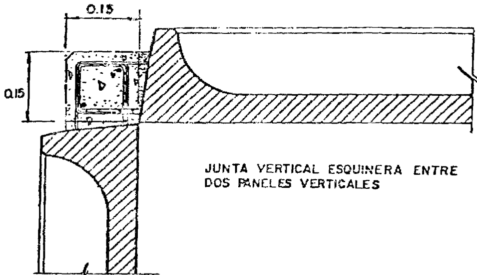
JUNTA VERTICAL ENTRE DOS PANELES VERTICALES
