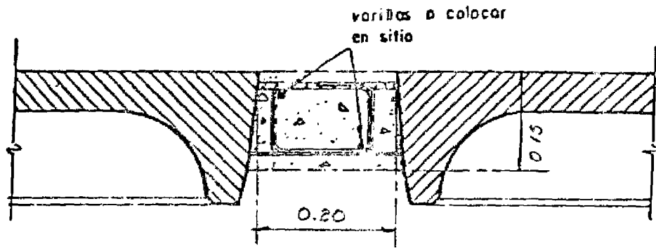
JUNTA VERTICAL ENTRE DOS PANELES VERTICALES
