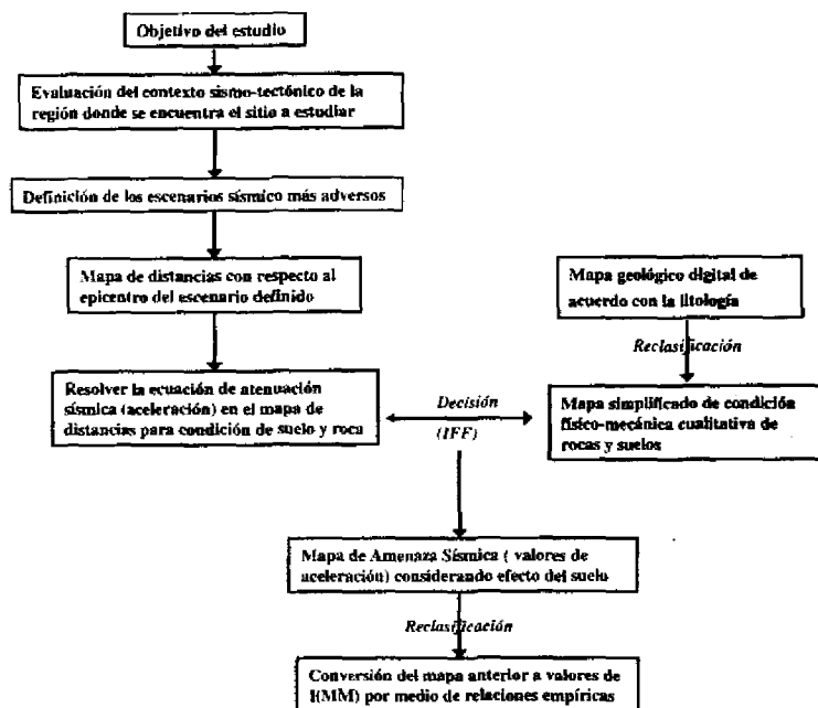
Fig. 5: Esquema simplificado para la estimación de la amenaza sísmica determinística utilizando un SIG.
