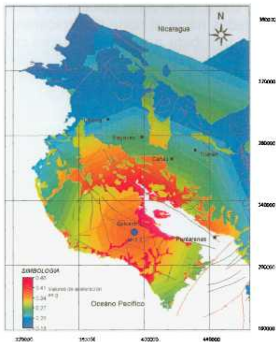
Fig. 6: Amenaza sísmica en la región noroeste de Costa Rica, dado que ocurre un sismo de magnitud 7,7 en la península de Nicoya y asociado a la subducción (Escenario 1).
