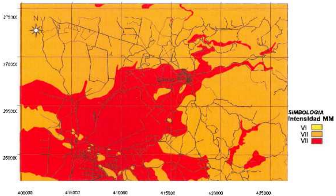
Fig. 9: Mapa de amenaza sísmica en valores de Intensidad MM en ciudad de Cañas de acuerdo al escenario sísmico 1.
