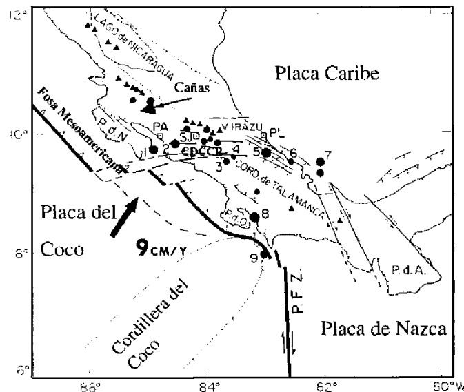
Fig. 2: Marco tectónico regional de Costa Rica (tomado de Jacob et al , 1991).
