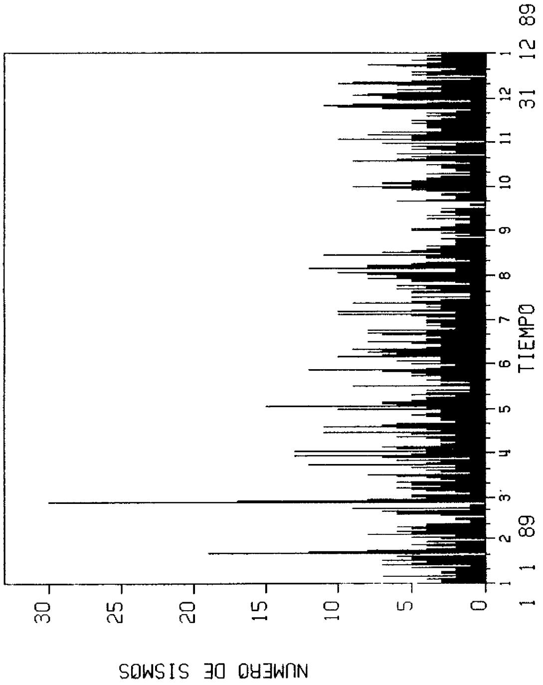
GRAFICO III-1 HISTOGRAMA DEL NUMERO DE EVENTOS POR DIA (TODAS MAGNITUDES. 1989)
